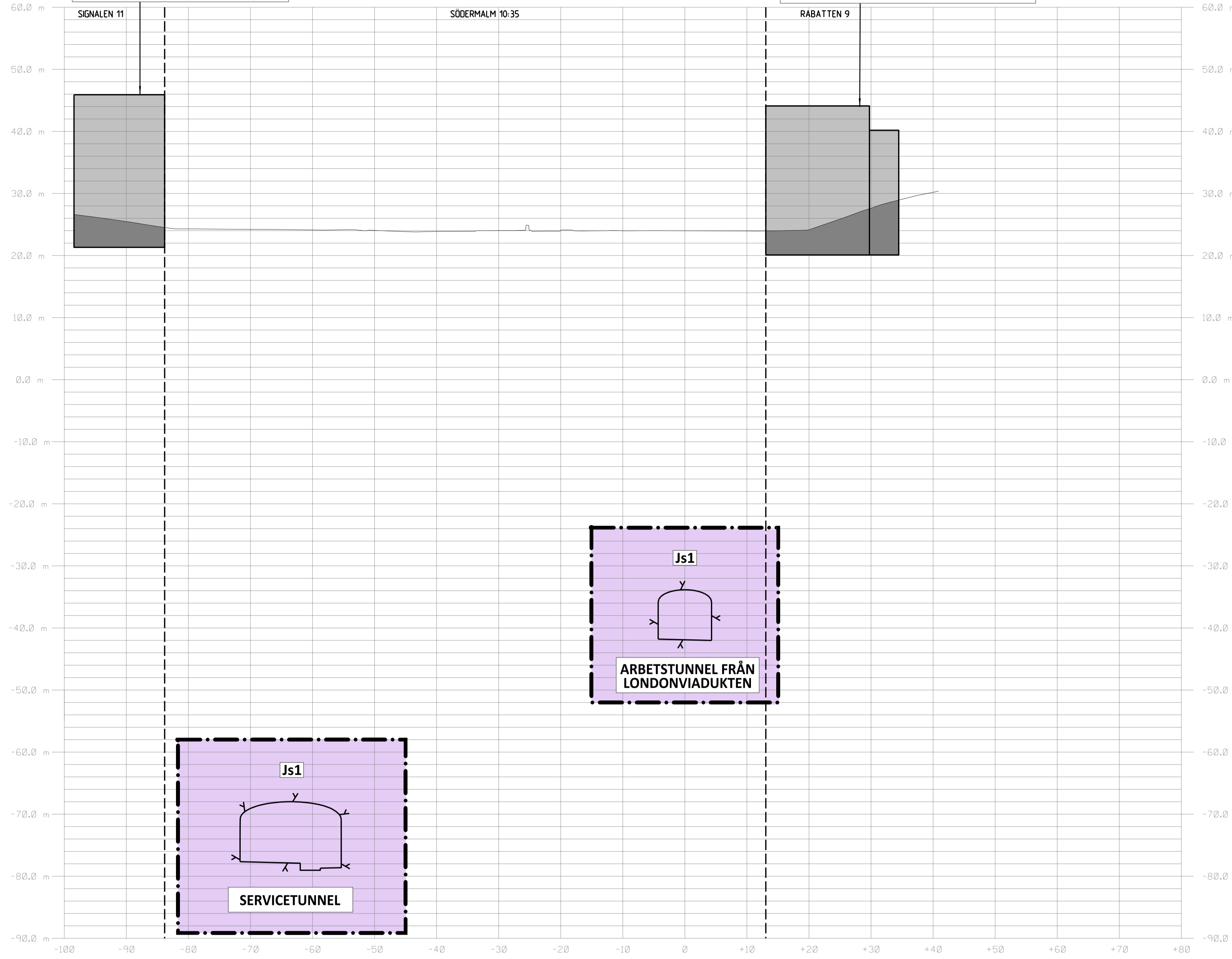
SEKTION S 1+955 SKALA 1:400
