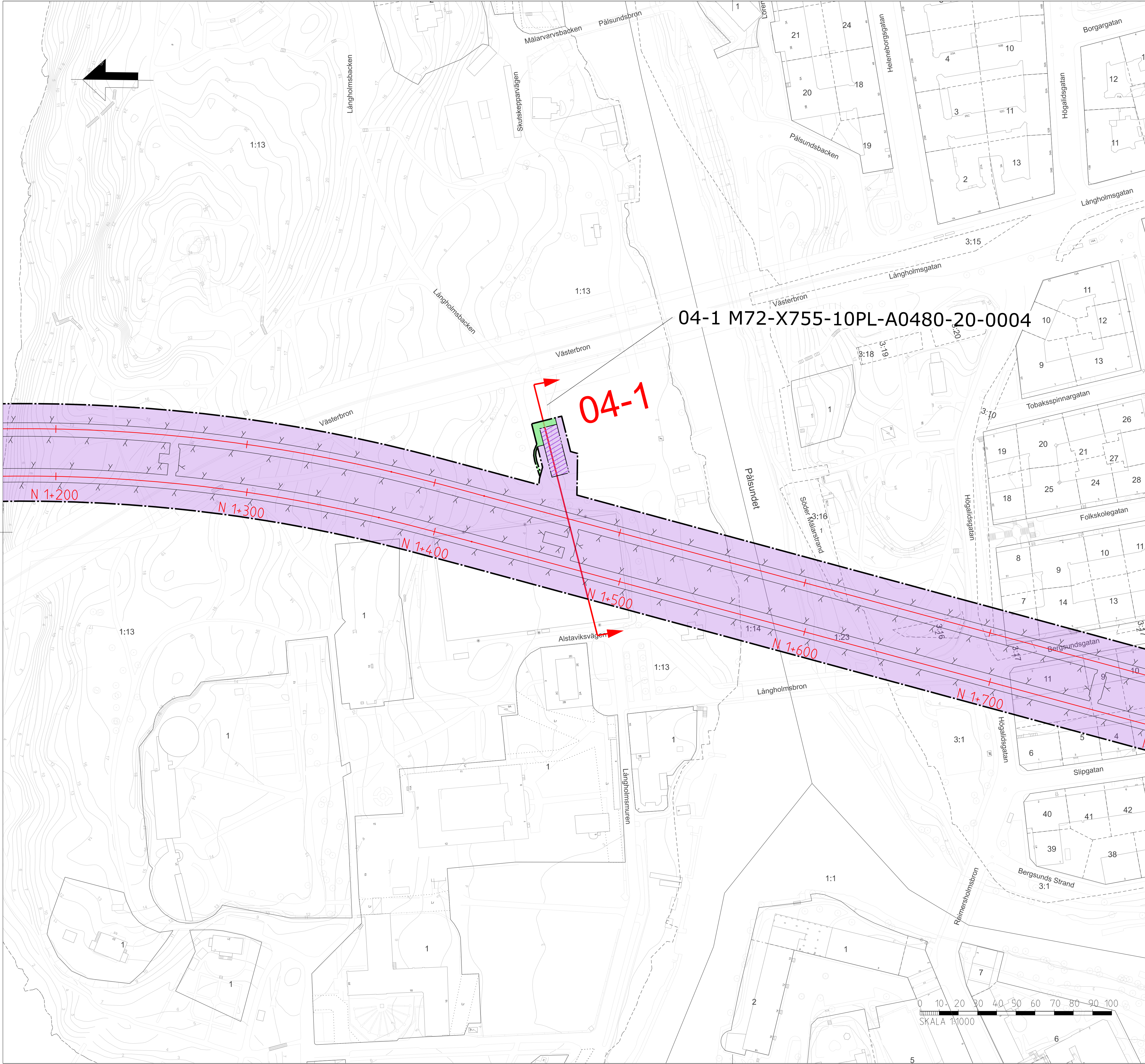
ÖVERSIKTSKARTA BLAD 04 Teknikbyggnad Översiktskarta sektionsmarkeringar för Permanent markanspråk
