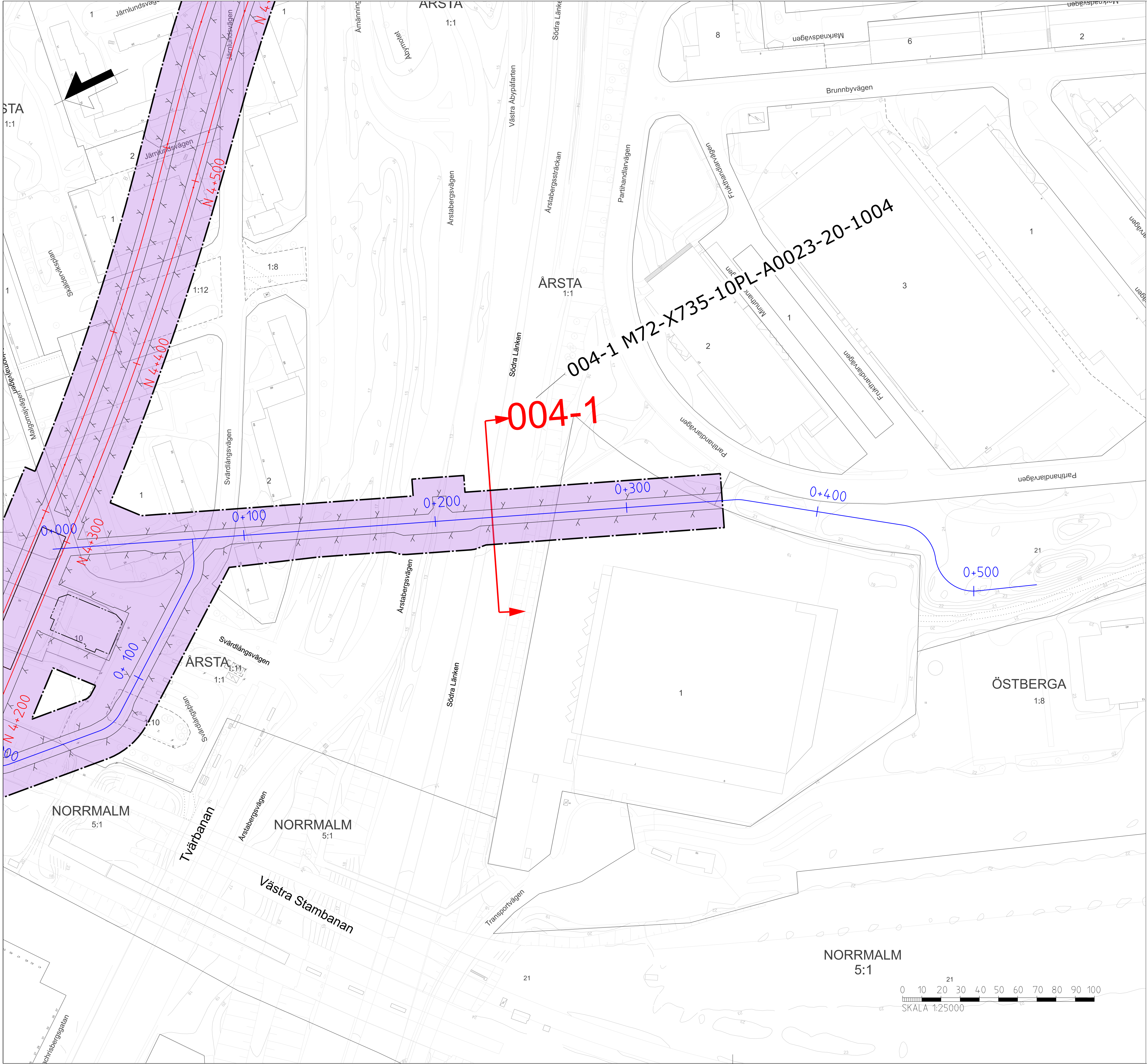
ÖVERSIKTSKARTA BLAD 004 Arbetstunnel Årstakrossen Översiktskarta sektionsmarkering för Permanent markanspråk
