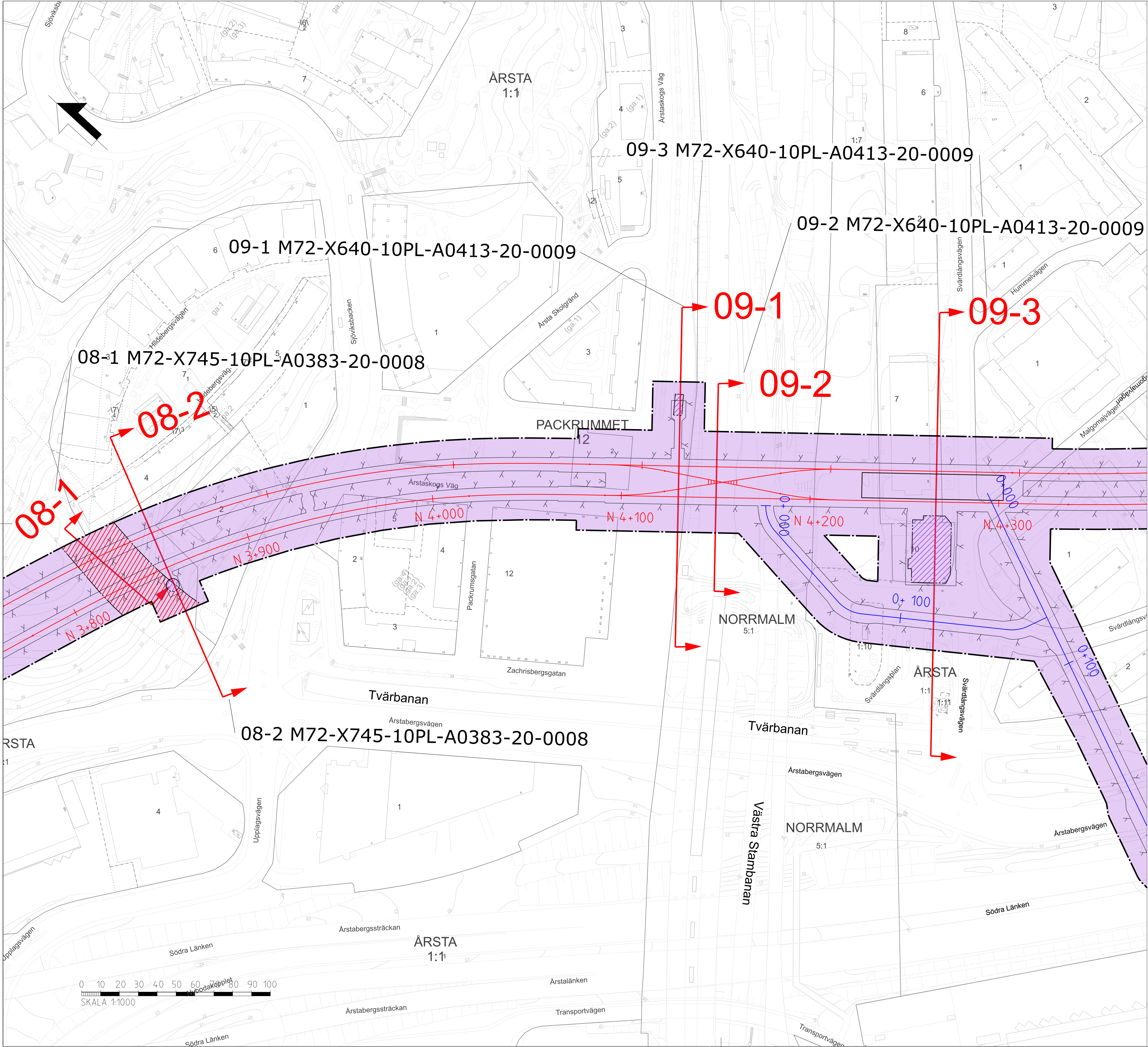
ÖVERSIKTSKARTA BLAD 08 OCH 09 Station Årstaberg Översiktskarta sektionsmarkering för Permanent markanspråk
