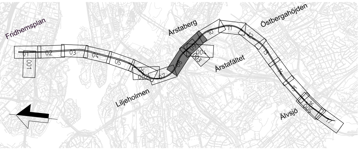
ÖVERSIKTSKARTA BLAD 08 OCH 09 Station Årstaberg Översiktskarta sektionsmarkering för Permanent markanspråk
