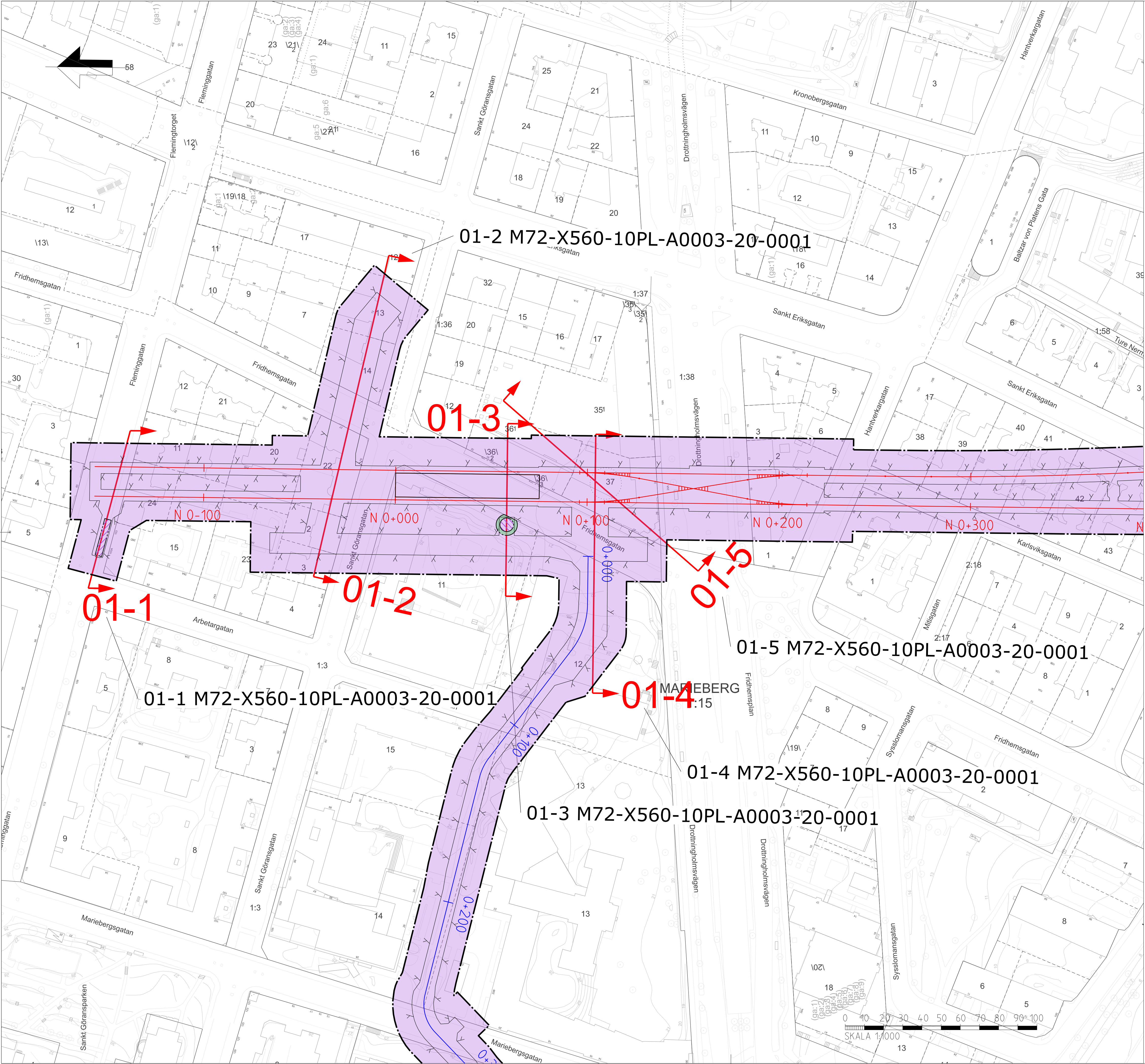
ÖVERSIKTSKARTA BLAD 01 Fridhemsgatan Översiktskarta sektionsmarkering för Permanent markanspråk
