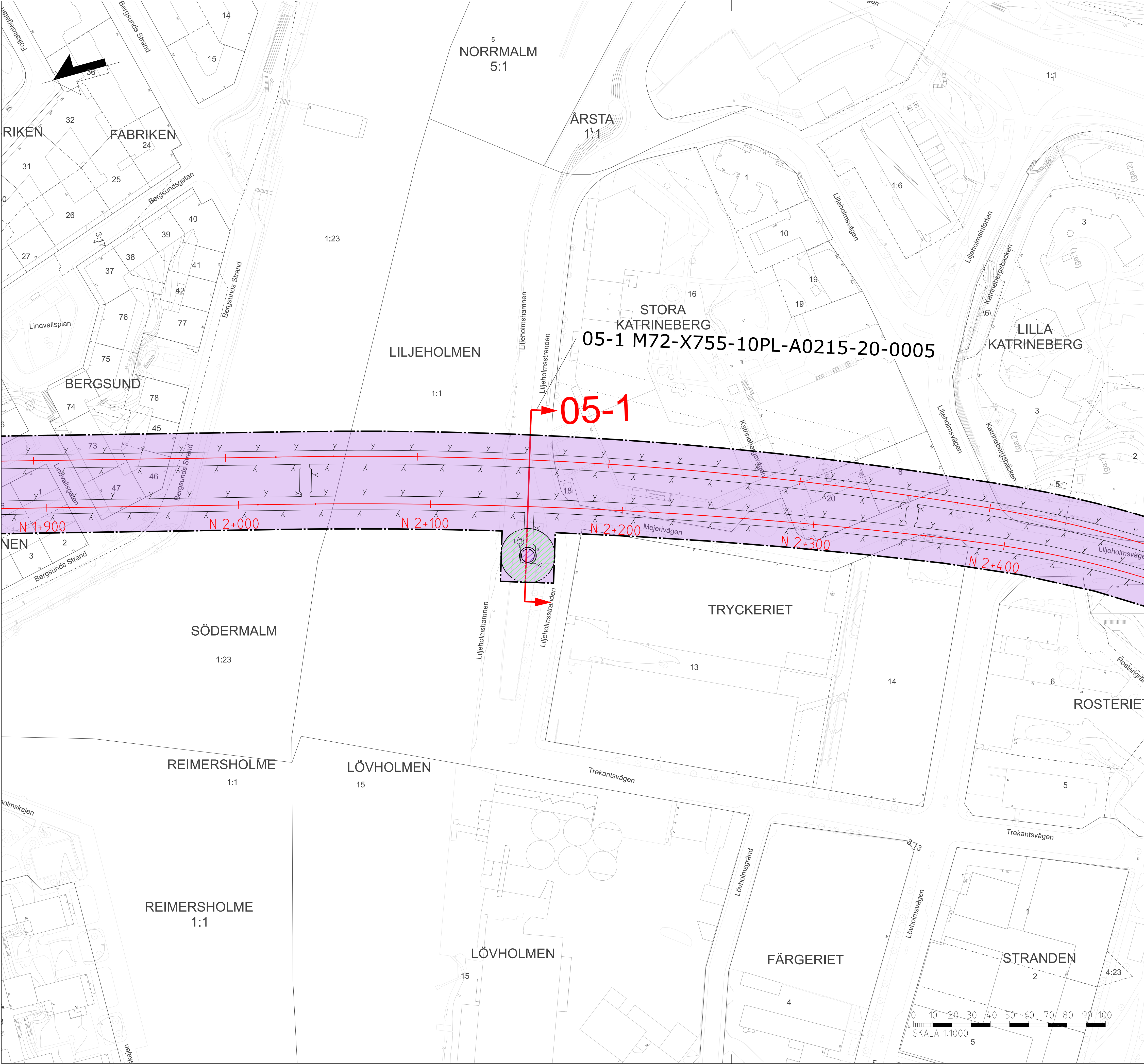
ÖVERSIKTS BLAD 05 Luftutbytesschakt Liljeholmsstranden Översiktsskarta sektionsmarkeringar för Permanent markanspråk
