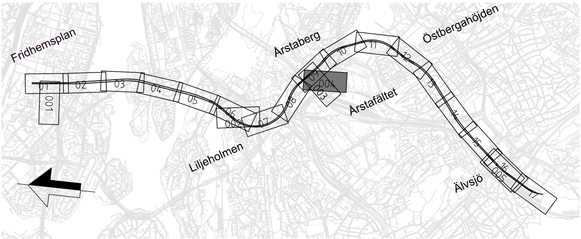
ÖVERSIKTSKARTA BLAD 004 Arbetstunnel Årstakrossen Översiktskarta sektionsmarkering för Permanent markanspråk
