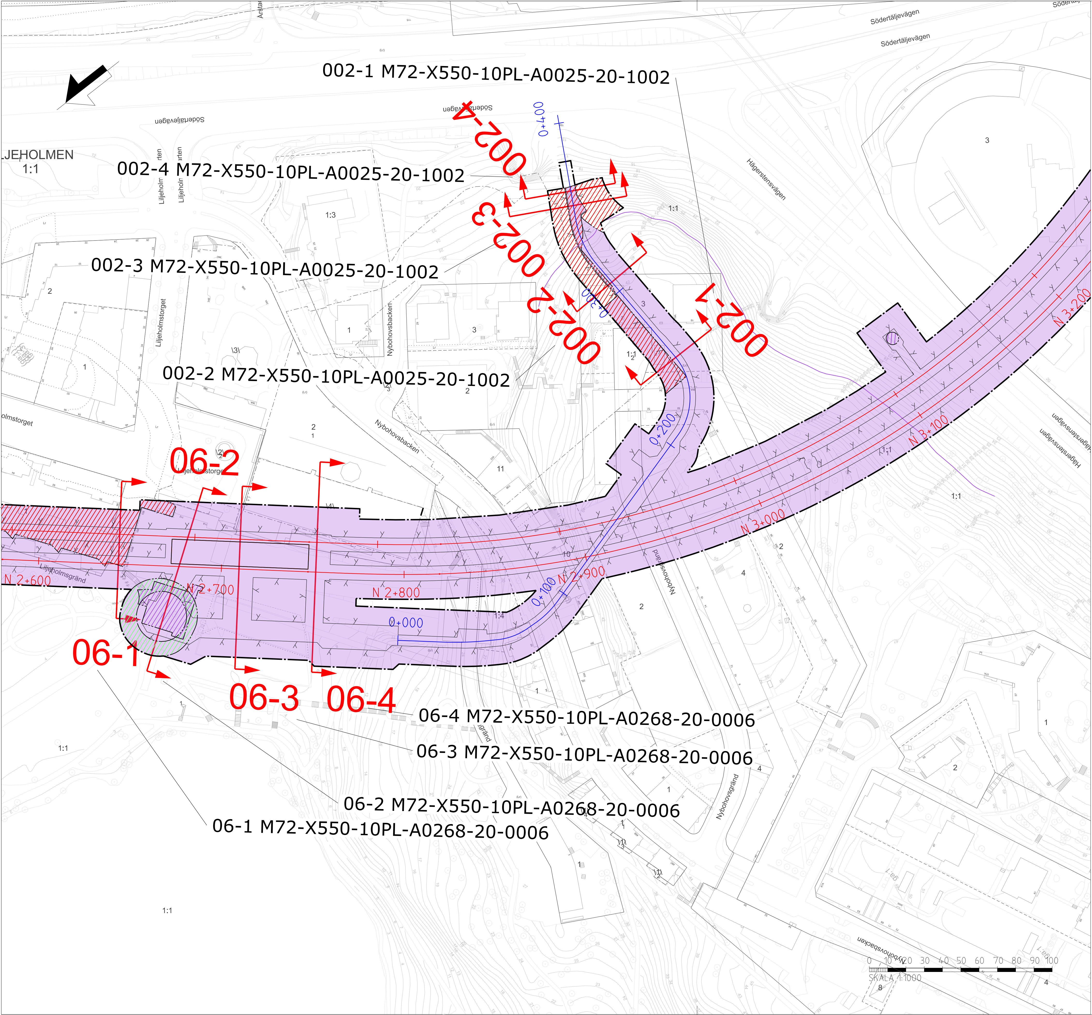
ÖVERSIKTSKARTA BLAD 06 OCH 002 Station Liljeholmen och Arbetstunnel Södertäljevägen Översiktskarta sektionsmarkeringar för Permanent markanspråk
