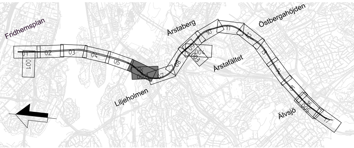
ÖVERSIKTSKARTA BLAD 06 OCH 002 Station Liljeholmen och Arbetstunnel Södertäljevägen Översiktskarta sektionsmarkeringar för Permanent markanspråk
