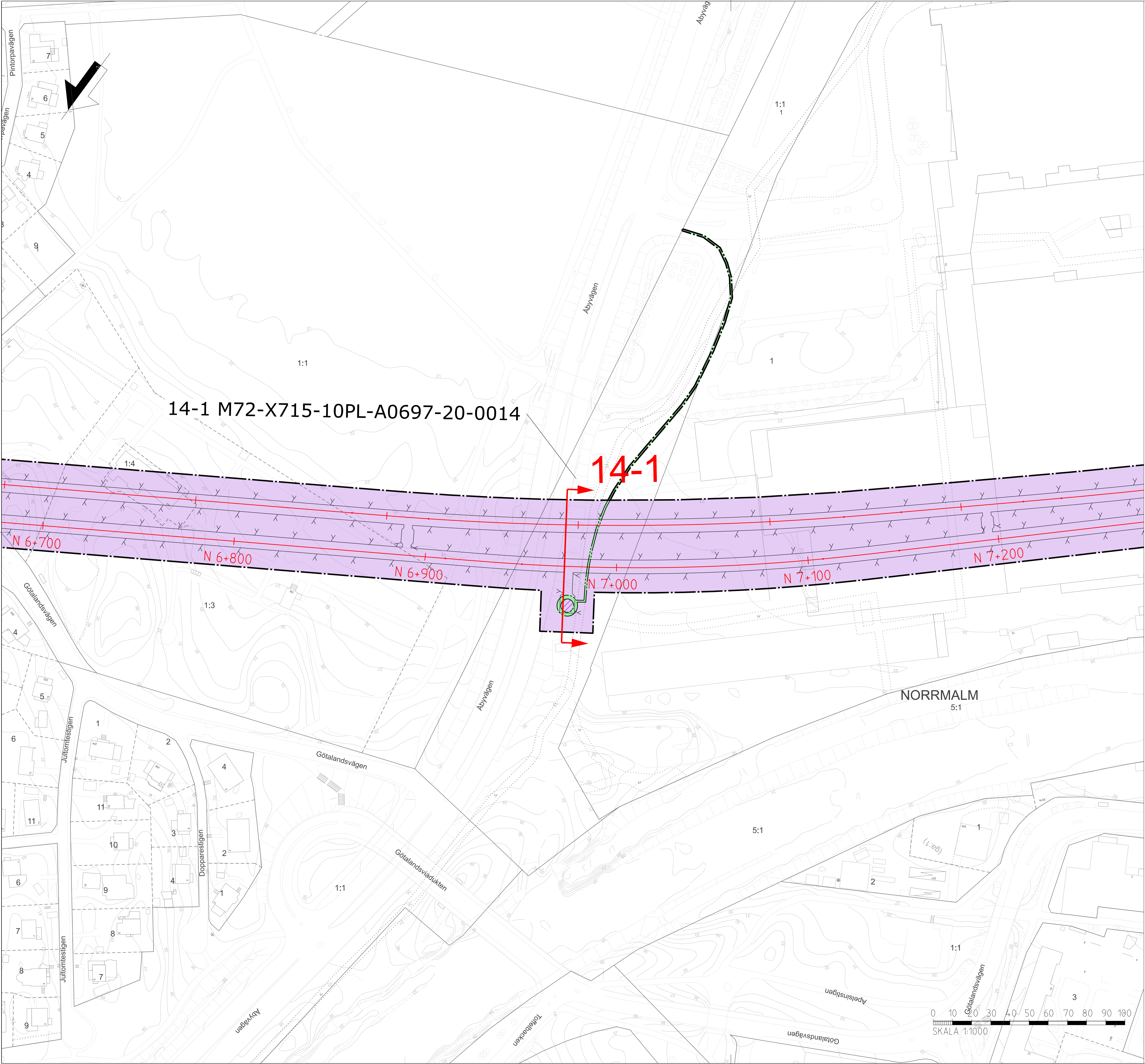
ÖVERSIKTSKARTA BLAD 14 Luftutbytesschakt Åbyvägen Översiktsskarta sektionsmarkering för Permanent markanspråk
