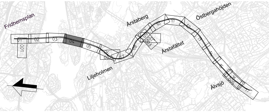
ÖVERSIKTSKARTA BLAD 04 Teknikbyggnad Översiktskarta sektionsmarkeringar för Permanent markanspråk
